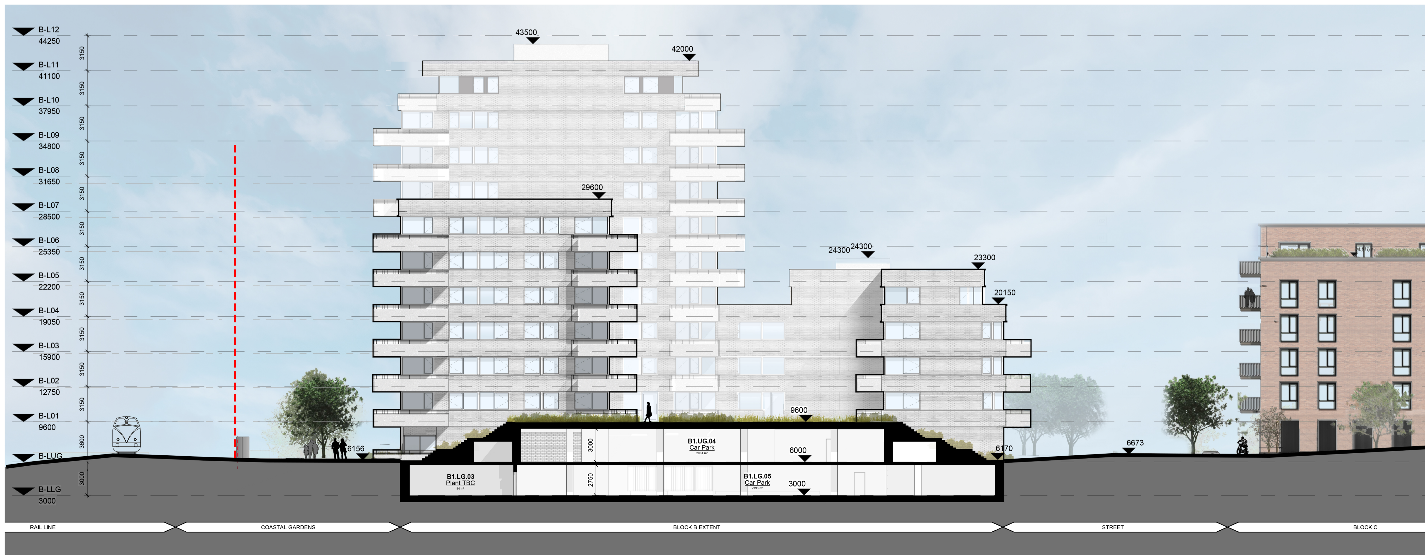
Block B - Section BB 1 : 200
